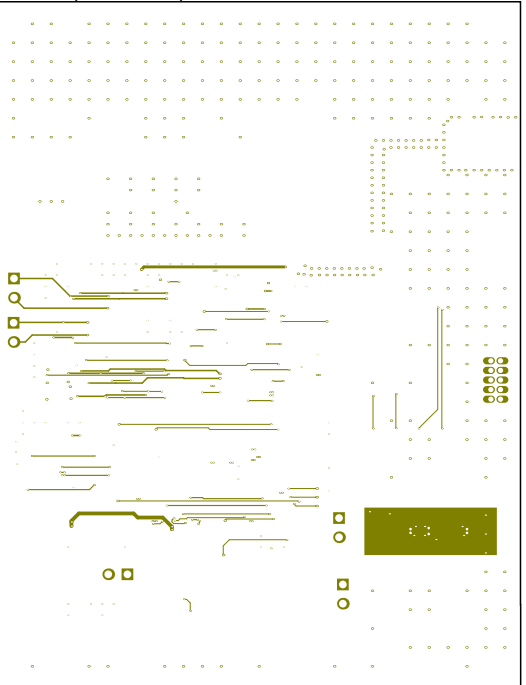
AHOR (Scale 1:1)
