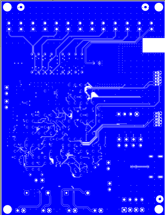
BOT (Scale 1:1)
